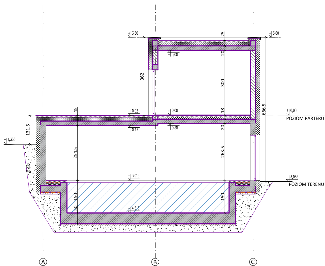
PRZEKRÓJ BB
